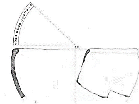
Pentola tipo 1
