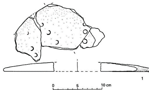
Coperchio tipo 1
