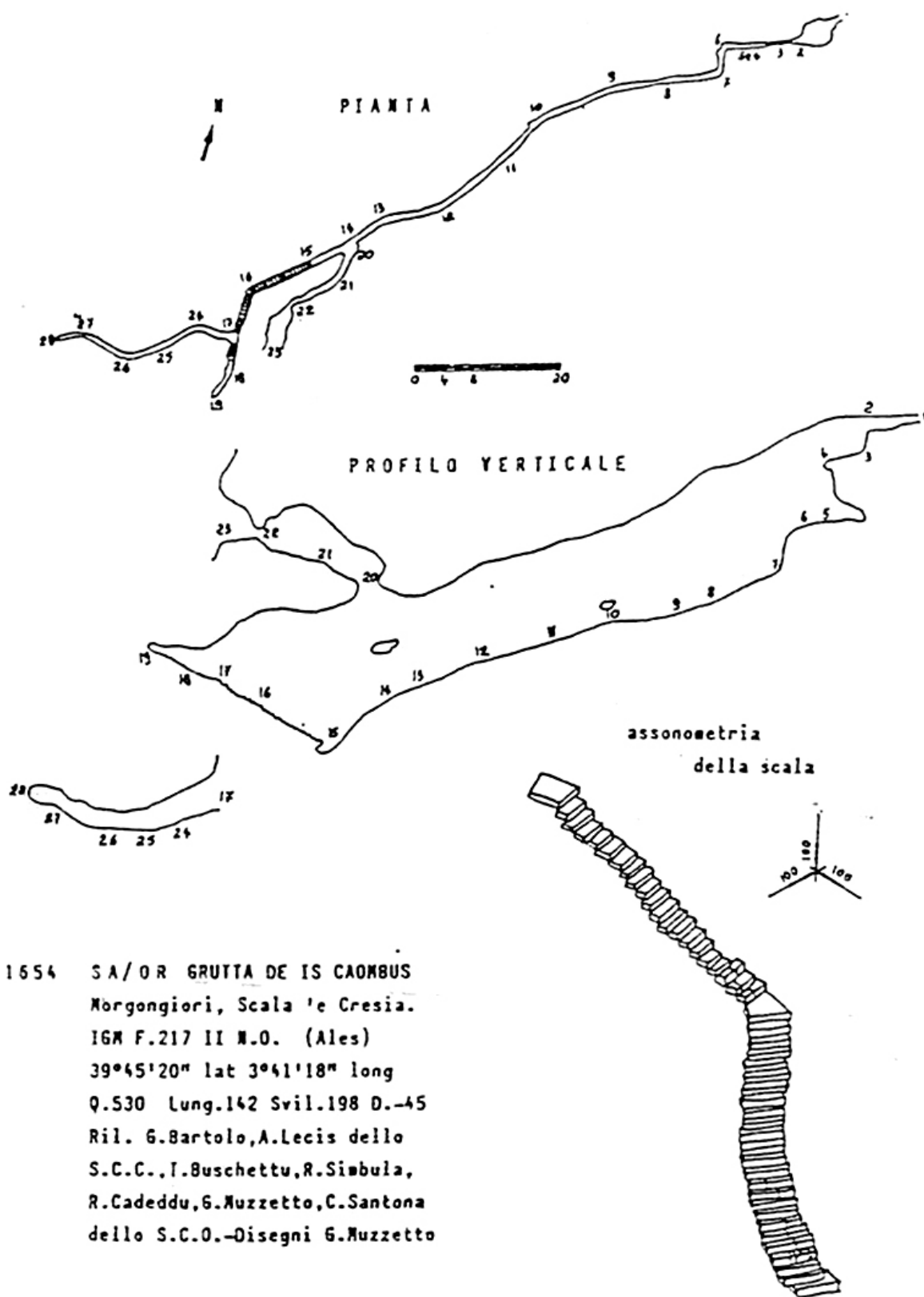
Fig. 3. Morgongiori, loc. Scala 'e Cresia. Rilievo planimetrico della grotta (da Lecis & Muzzetto, 1989).
