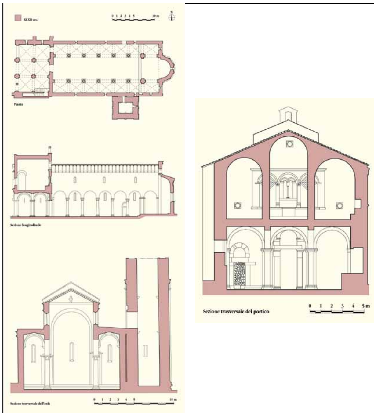
Fig. 2. Ozieri, Sant'Antioco di Bisarcio, rilievi (da Coroneo, 1993).
